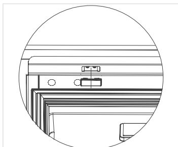
Төменгі шектегіштерге бітеуіштерді орнатыңыз
